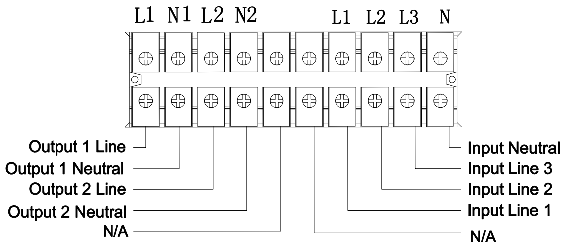
Клеммная панель моделей 15кВА / 20кВА
