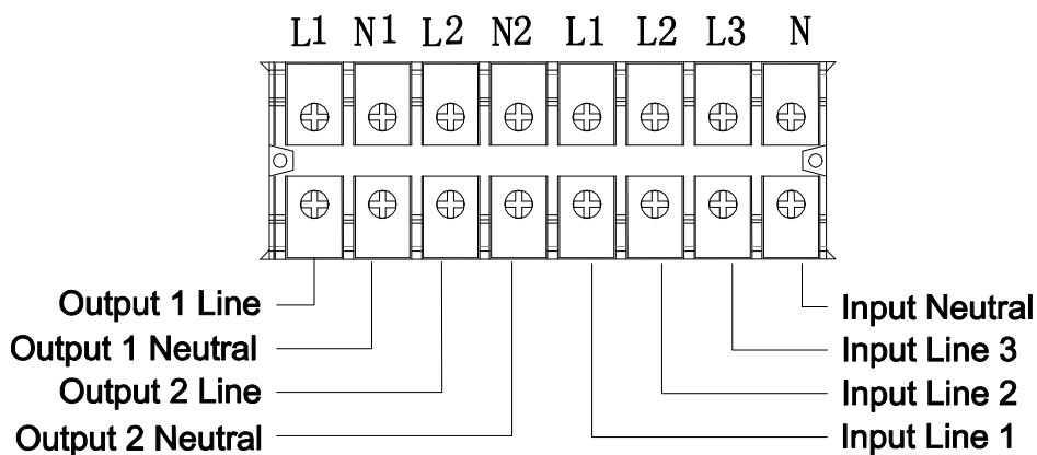
Клеммная панель моделей 10кВА (LT)
