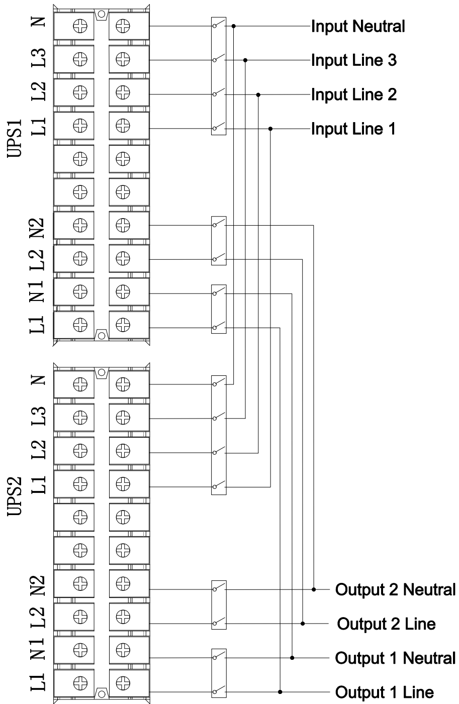
Схема подключения параллельной системы из 2х ИБП Grand-Vision 15кВА (LT) / 20кВА (LT)
