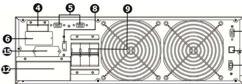
Grand-Vision 10кВА RM (LT), обратная сторона.
