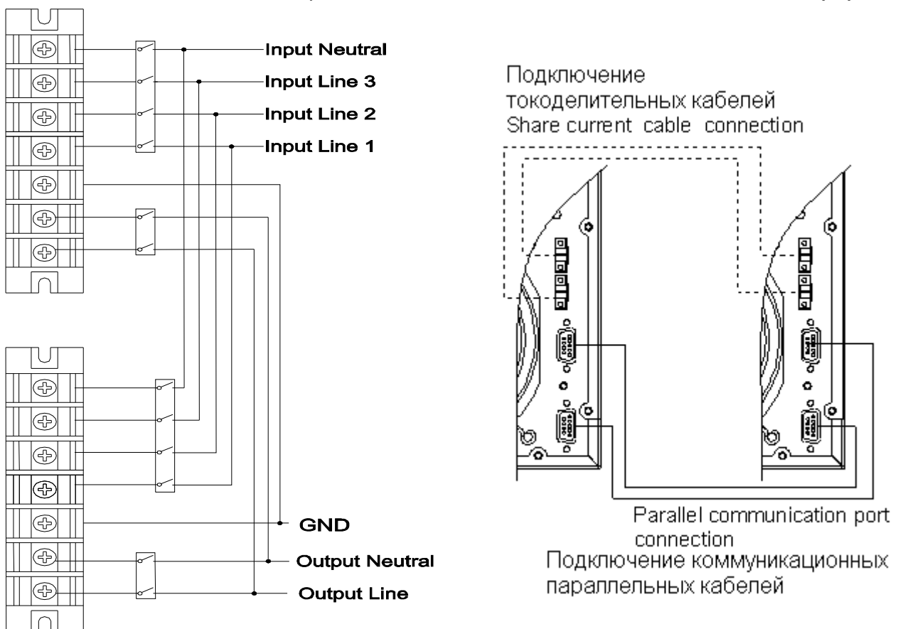
Схема подключения параллельной системы из 2х ИБП Grand-Vision 15кВА RM (LT) / 20кВА RM (LT)
