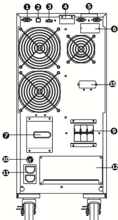
Grand-Vision 10кВА (LT), обратная сторона.
