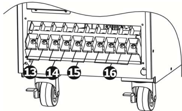
Grand-Vision 15кВА LT / 20кВА LT ВХОДНАЯ / ВЫХОДНАЯ клеммная панель
