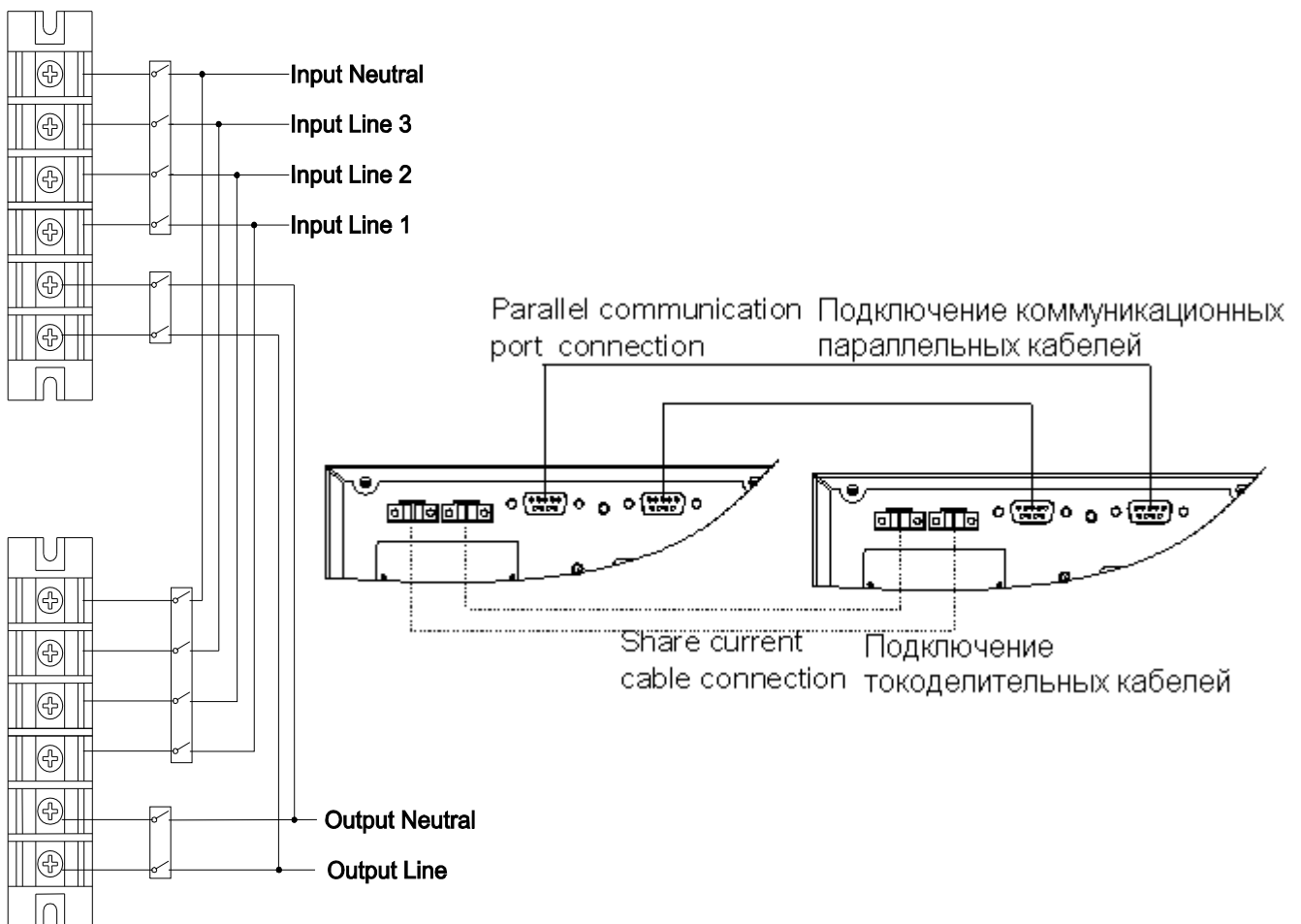
Схема подключения параллельной системы из 2х ИБП Grand-Vision 10кВА RM (LT)
