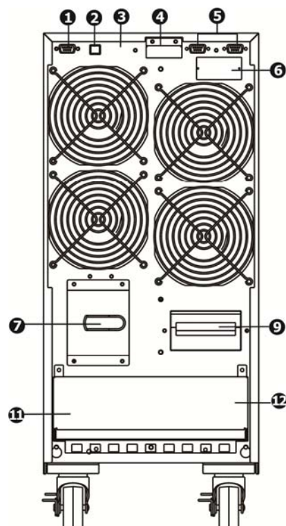
Grand-Vision 15кВА LT/20кВА LT, обратная сторона.
