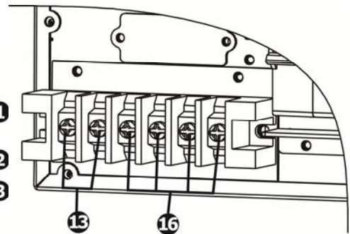
Grand-Vision 10кВА RM (LT), ВХОДНАЯ / ВЫХОДНАЯ клеммная панель
