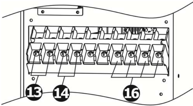
Grand-Vision 15кВА / 20кВА ВХОДНАЯ / ВЫХОДНАЯ клеммная панель
