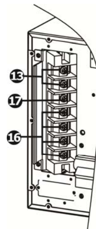
Grand-Vision 15кВА RM(LT)/20кВА RM(LT), ВХОДНАЯ / ВЫХОДНАЯ клеммная панель
