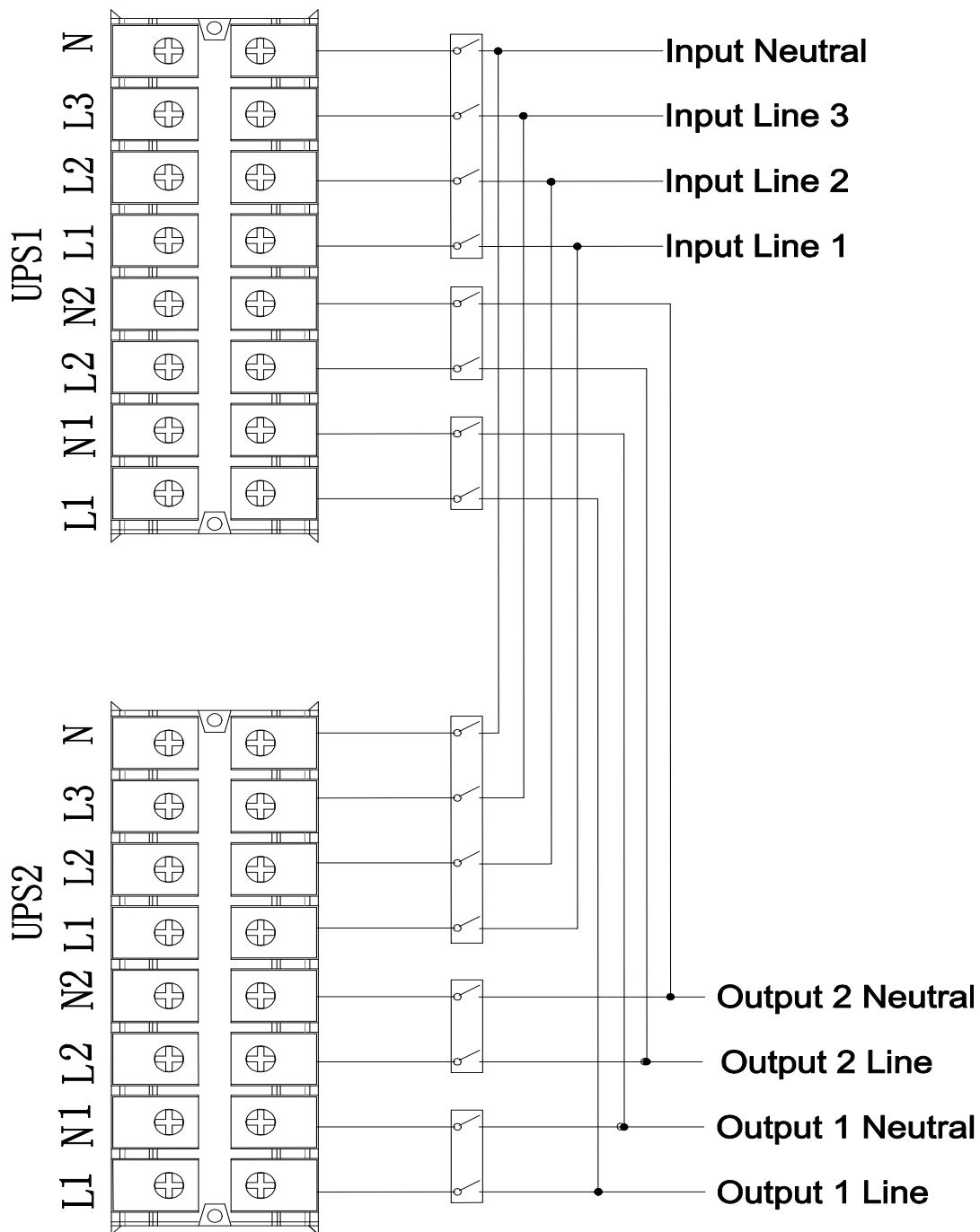
Схема подключения параллельной системы из 2х ИБП Grand-Vision 10кВА(LT)
