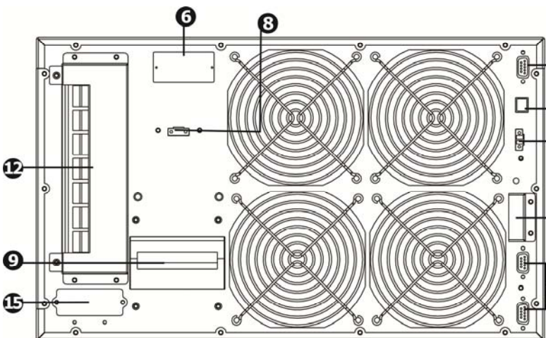
Grand-Vision 15кВА RM(LT)/20кВА RM(LT), обратная сторона.
