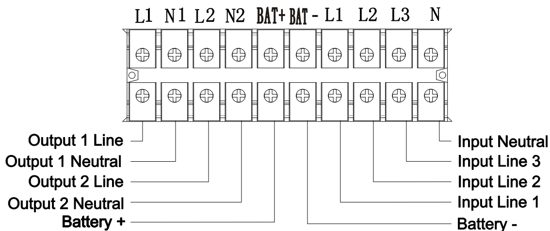
Клеммная панель моделей 15кВА LT / 20кВА LT
