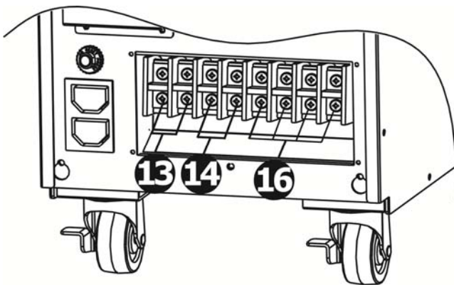
Grand-Vision 10кВА(LT) ВХОДНАЯ / ВЫХОДНАЯ клеммная панель
